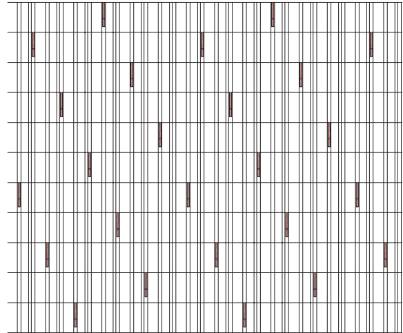
29. Minden hatodik cserépbe akasztott hófogó (kb. 1,7–1,8 db / m 2 )
