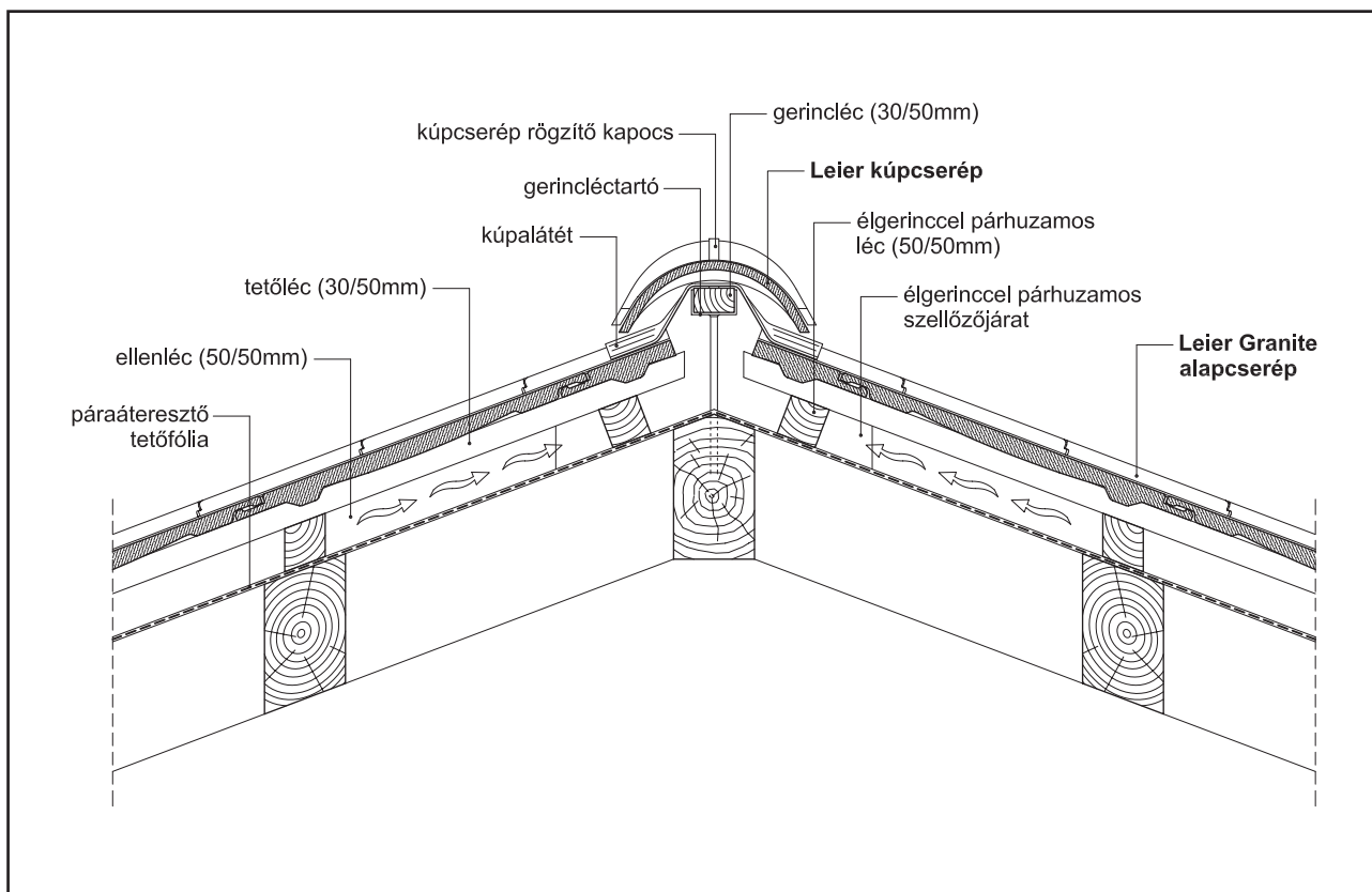
9/12 Élgerinc részlet Leier Granite 1:10
