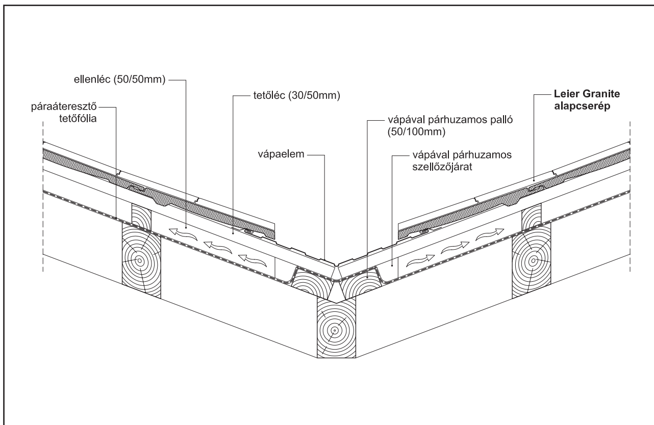
10/12 Vápa részlet Leier Granite 1:10
