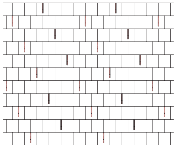
31. Minden hatodik cserépbe akasztott hófogó (kb. 1,7–1,8 db / m 2 )
