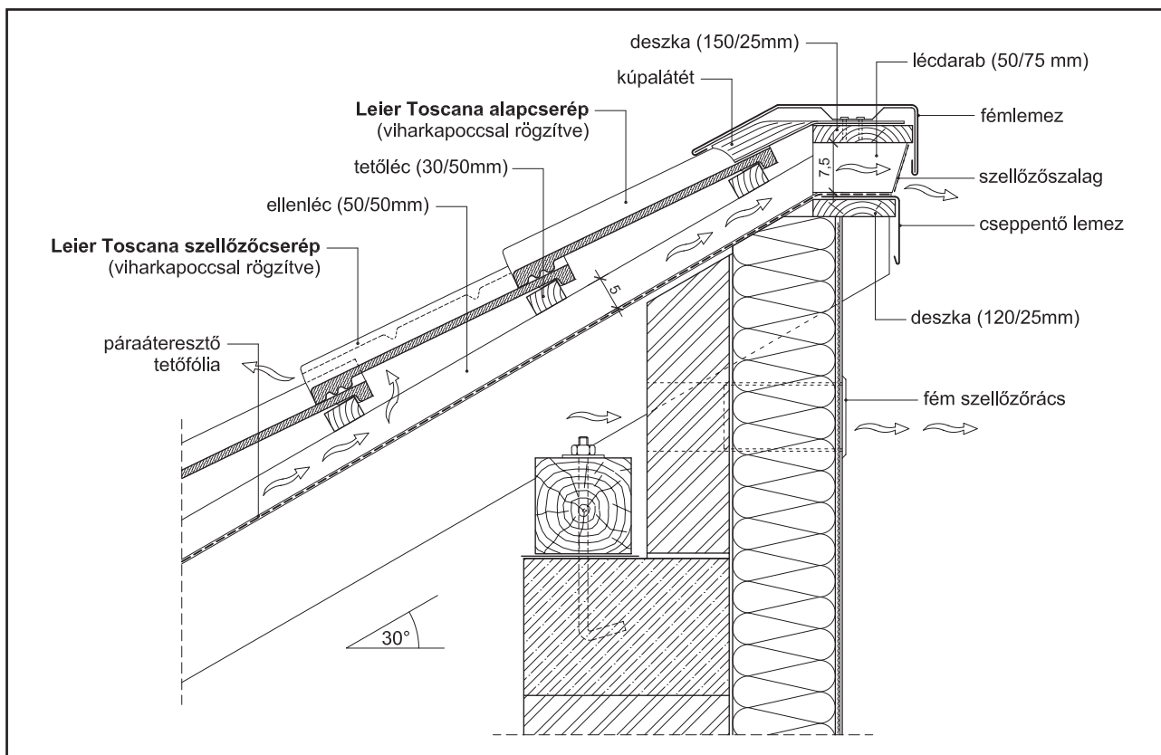
6/12 Félnyereg gerinc részlet Leier Toscana 1:10
