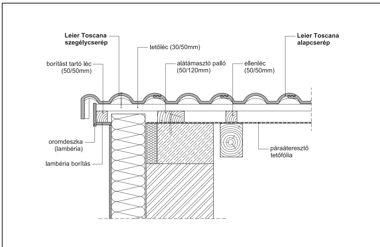
5/12 Oromszegély részlet Leier Toscana 1:10
