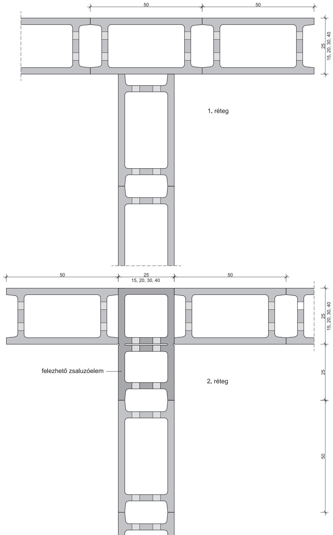
21. Falcsatlakozás: Leier beton zsaluzóelem (ZS 15, ZS 20, ZS 25, ZS 30, ZS 40)
