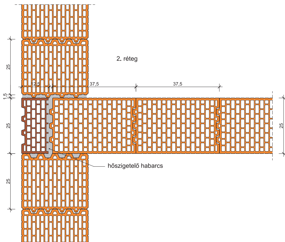
70. FalcSATlakozás: LeierPLAN 30 Pro – LeierPLAN 25 N+F / LeierPLAN 30 N+F – LeierPLAN 25 N+F Leiertherm 30 Pro – Leiertherm 25 N+F / Leiertherm 30 N+F – Leiertherm 25 N+F
