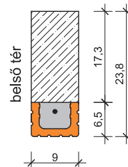
19. Leier MDA nyílásáthidaló elhelyezési lehetőségei
