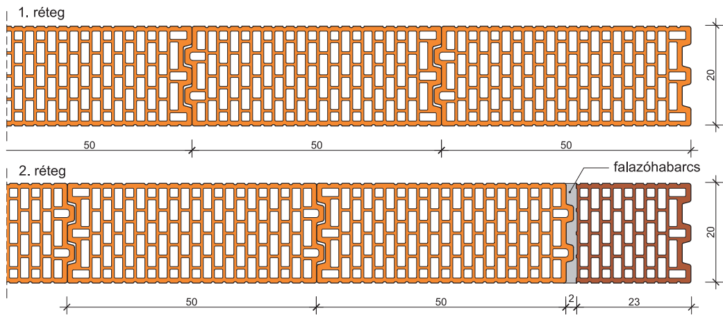
53. Falvég: Leiertherm 20 N+F
