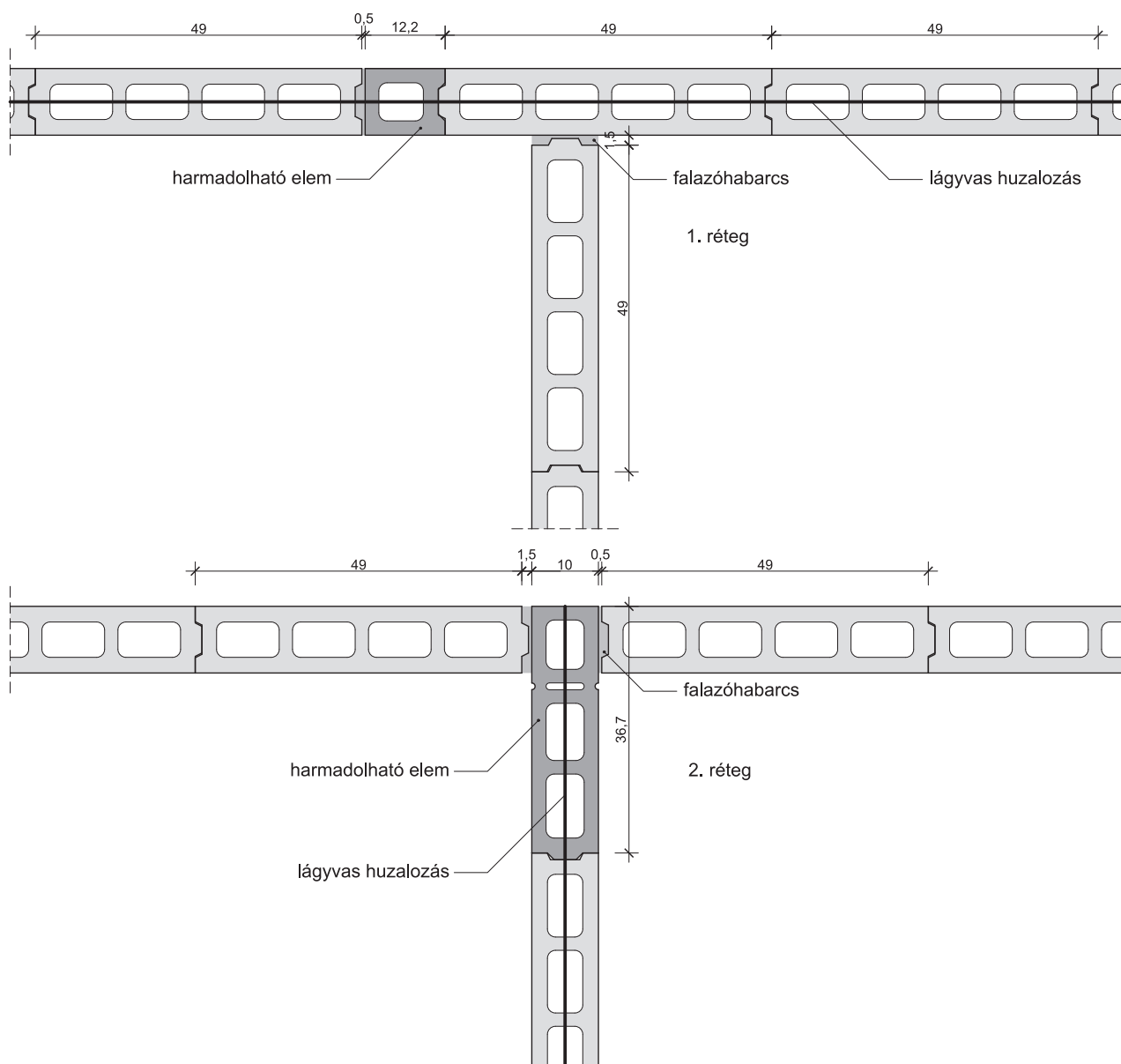
19. Falsarok: Leier beton válaszfalelem VF 10
