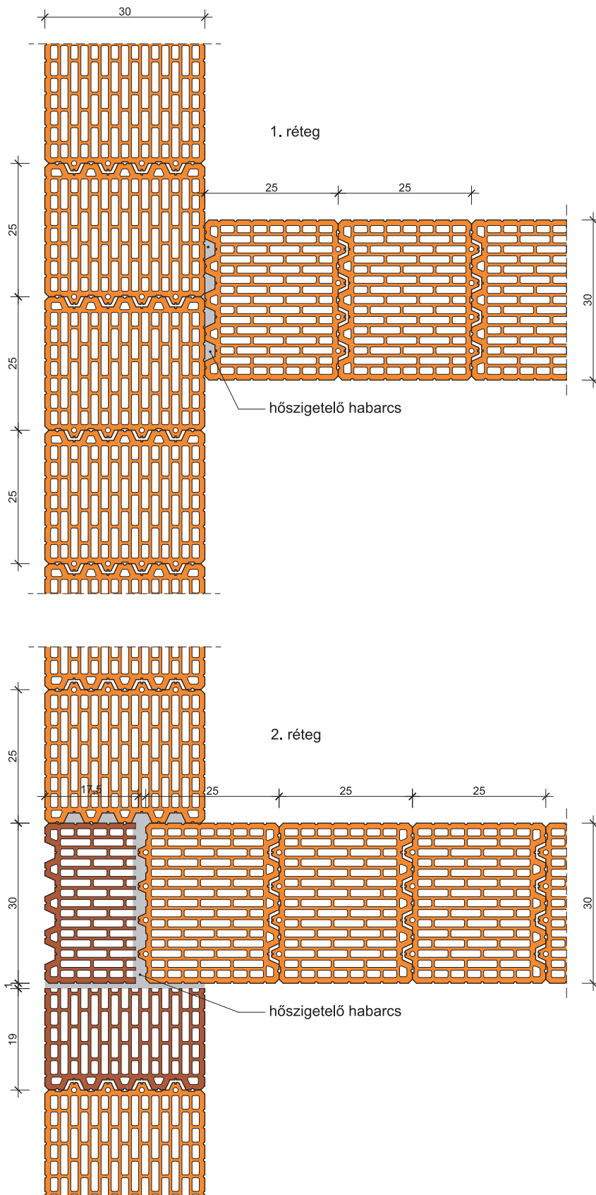
71. Falcsatlakozás: LeierPLAN 30 Pro – LeierPLAN 30 Pro / LeierPLAN 30 N+F – LeierPLAN 30 N+F Leiertherm 30 Pro – Leiertherm 30 Pro / Leiertherm 30 N+F – Leiertherm 30 N+F
