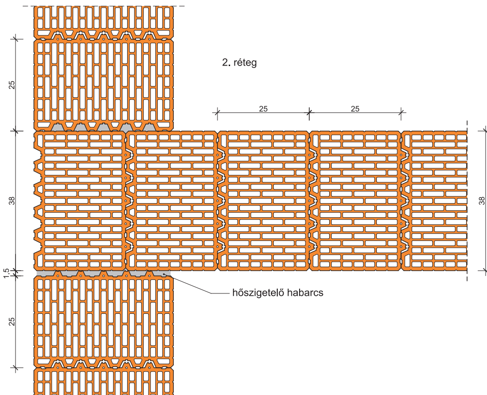
75. Falcsatlakozás: LeierPLAN 38 Pro – LeierPLAN 38 Pro / LeierPLAN 38 N+F – LeierPLAN 38 N+F Leiertherm 38 Pro – Leiertherm 38 Pro / Leiertherm 38 N+F – Leiertherm 38 N+F
