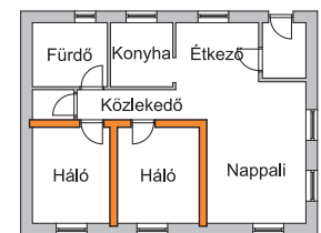
29. Nyugodt és zajos zónát elválasztó falak
