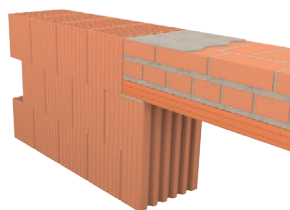
17. Leier MDA nyílásáthidaló beépítése
