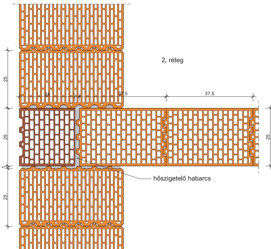
76. Falcsatlakozás: Leiertherm 45 N+F – Leiertherm 25 N+F
