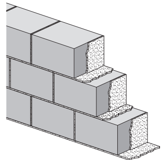
1. Habarcsréteg beton falszerkezetekben
