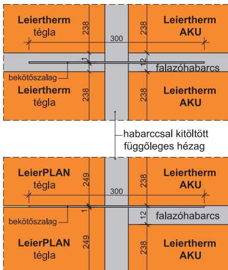
30. Bekötőszalag helye a fugában
