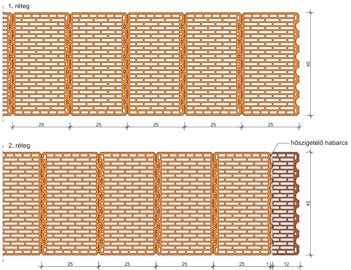
57. Falvég: LeierPLAN 45 N+F / Leiertherm 45 N+F
