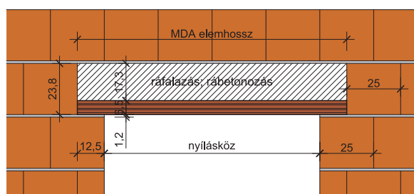
13. Leier MDA nyílásáthidaló oldalnézet
