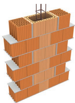
23. Leiertherm 30 U elemből készített falközi pillér - téglakötésben rakva
