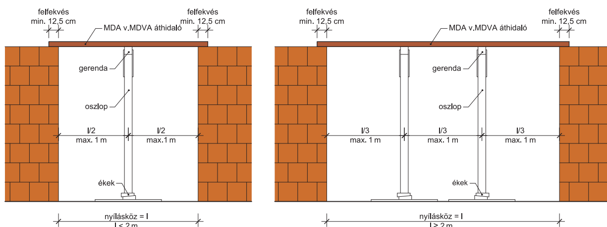
18. Leier MDA és Leier MDVA nyílásáthidalók ideiglenes alátámasztása a nyílásköz méretének függvényében
