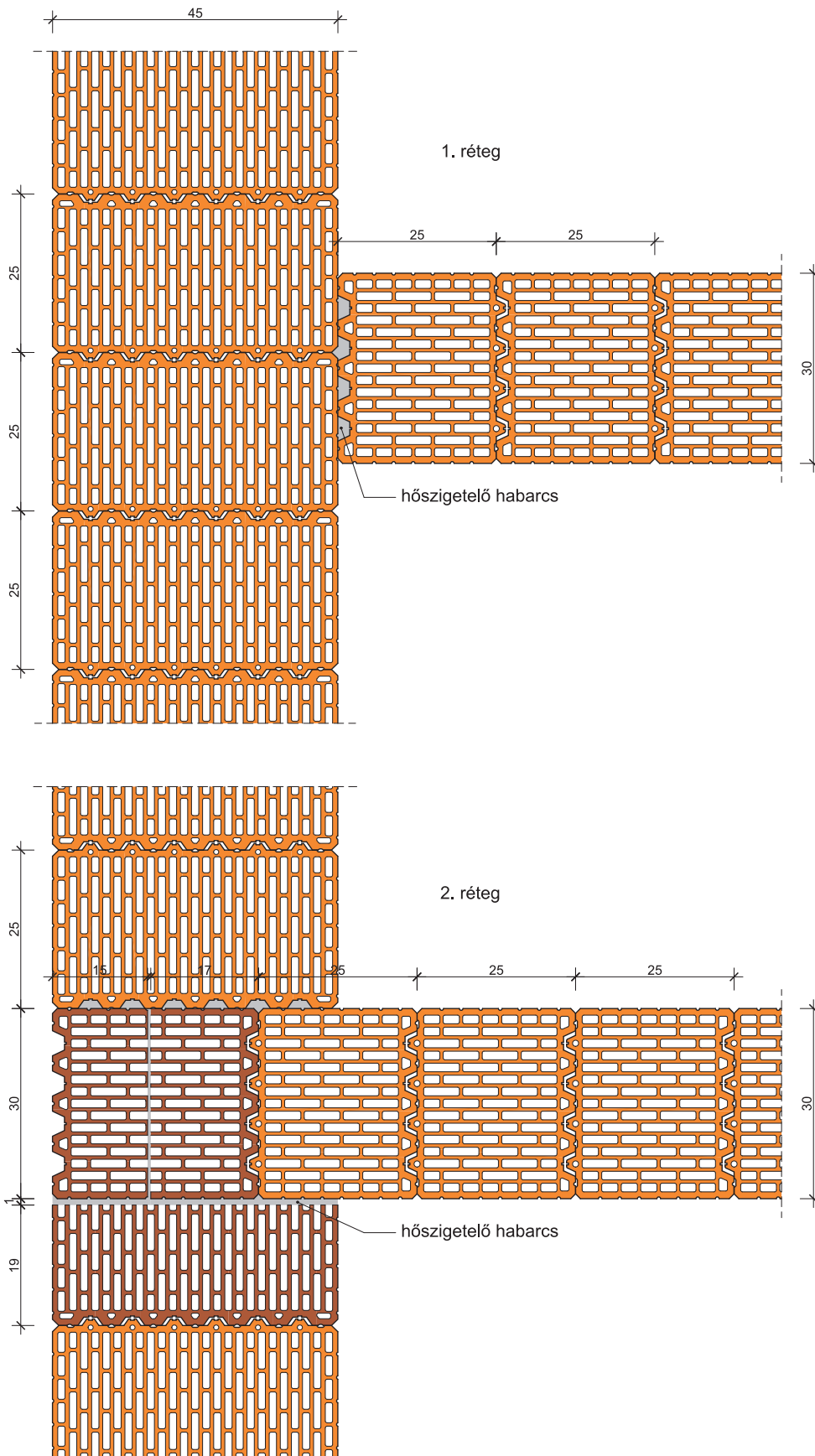
77. Falcsatlakozás: Leiertherm 45 N+F – Leiertherm 30 Pro / Leiertherm 45 N+F – Leiertherm 30 N+F
