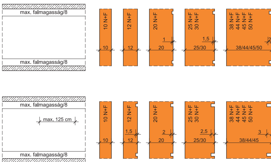
9. Vízszintes falhorony legnagyobb mérete (tetszőleges horonyhossz és max. 125 mm horonyhossz esetén)
