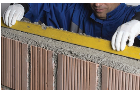
38. Hanggátló fal építése: falegyen képzés (25/30 AKU)
