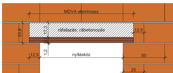
16. Leier MDVA nyílásáthidaló oldalnézet
