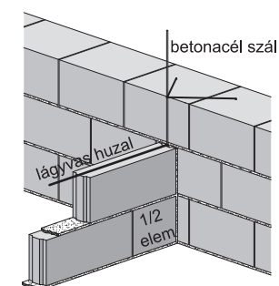
2. Beton válaszfal csatlakozása főfalhoz
