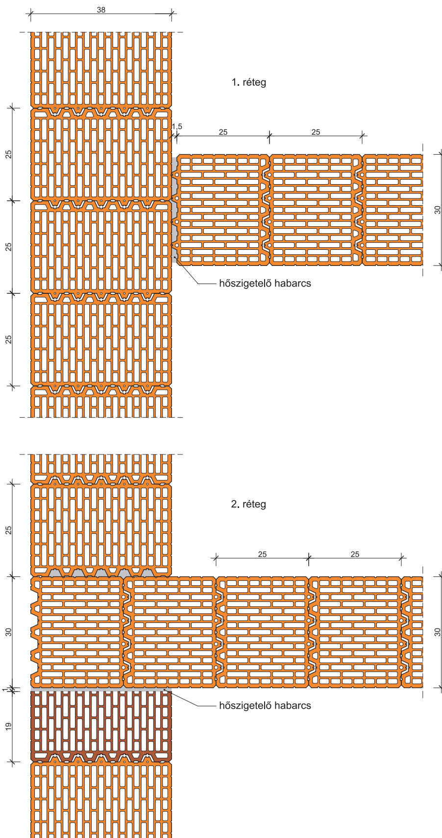
74. Falcsatlakozás: LeierPLAN 38 Pro – LeierPLAN 30 Pro / LeierPLAN 38 N+F – LeierPLAN 30 N+F Leiertherm 38 Pro – Leiertherm 30 Pro / Leiertherm 38 N+F – Leiertherm 30 N+F
