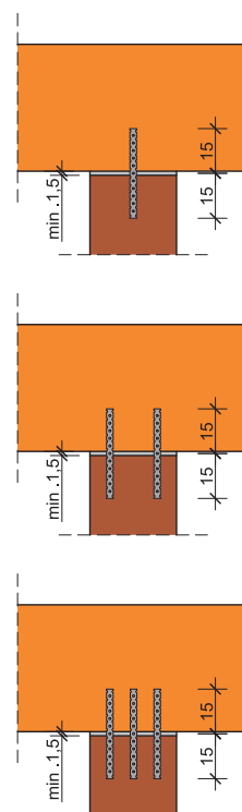
3. Egy, kettő és három bekötőszalag elhelyezése
