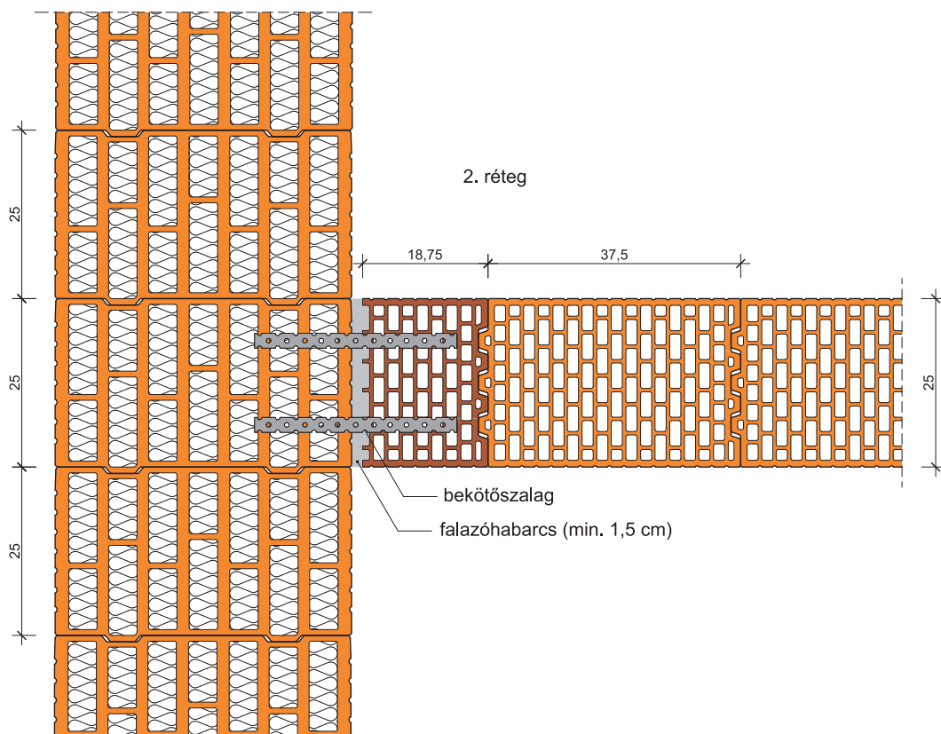
78. Falcsatlakozás: LeierPLAN 44 ISO – LeierPLAN 25 N+F
