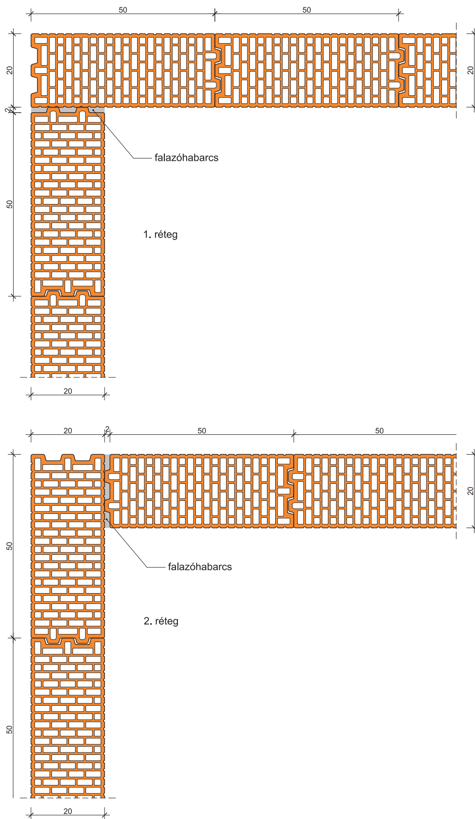
60. Falsarok: Leiertherm 20 N+F
