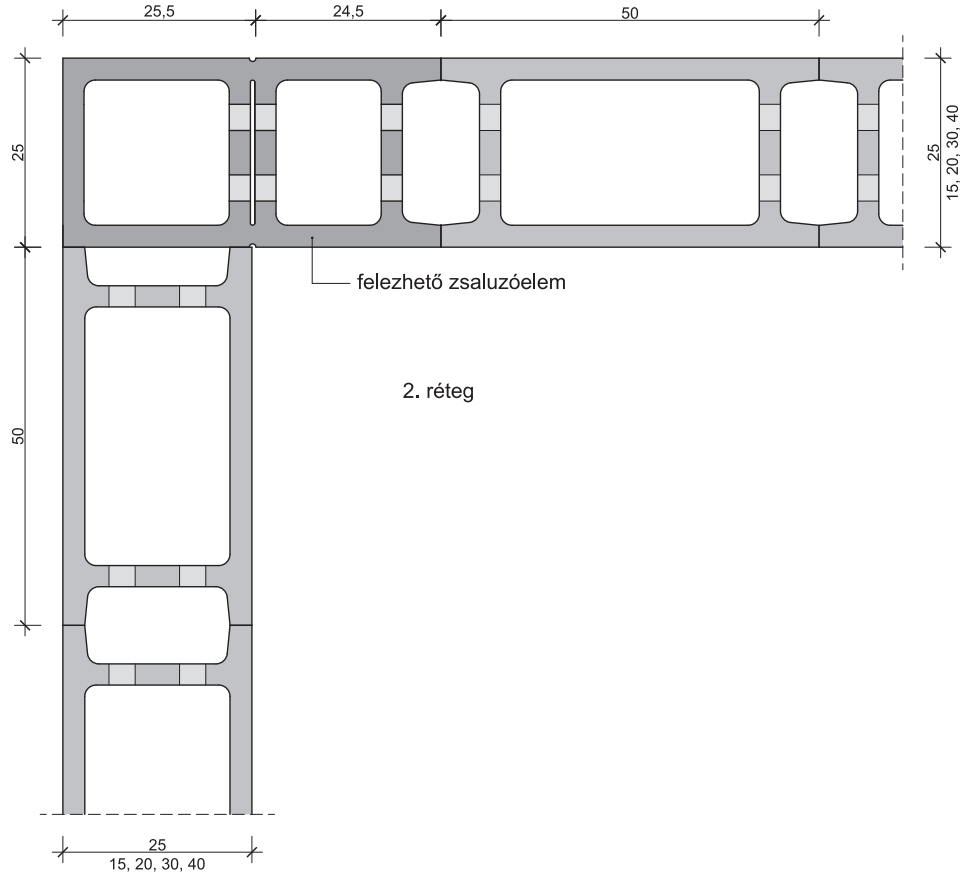
20. Falsarok: Leier beton zsaluzóelem (ZS 15, ZS 20, ZS 25, ZS 30, ZS 40)
