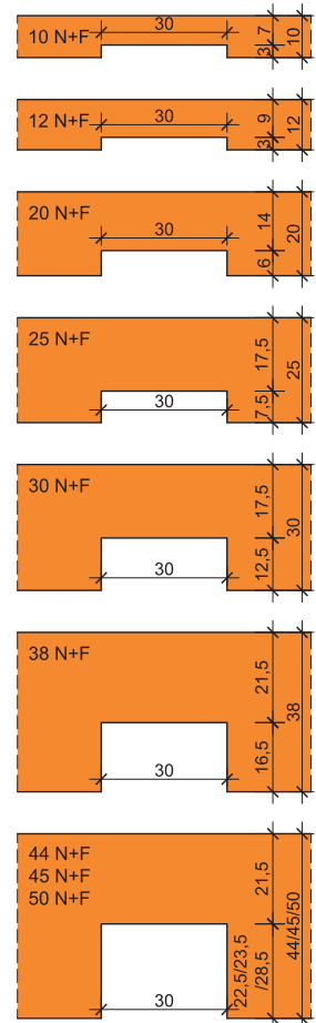
7. Függőleges falhorony legnagyobb mérete új építésű fal esetén
