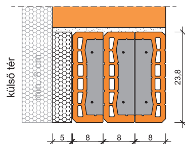
10. Leier MDE nyílászáró elhelyezési lehetőségei
