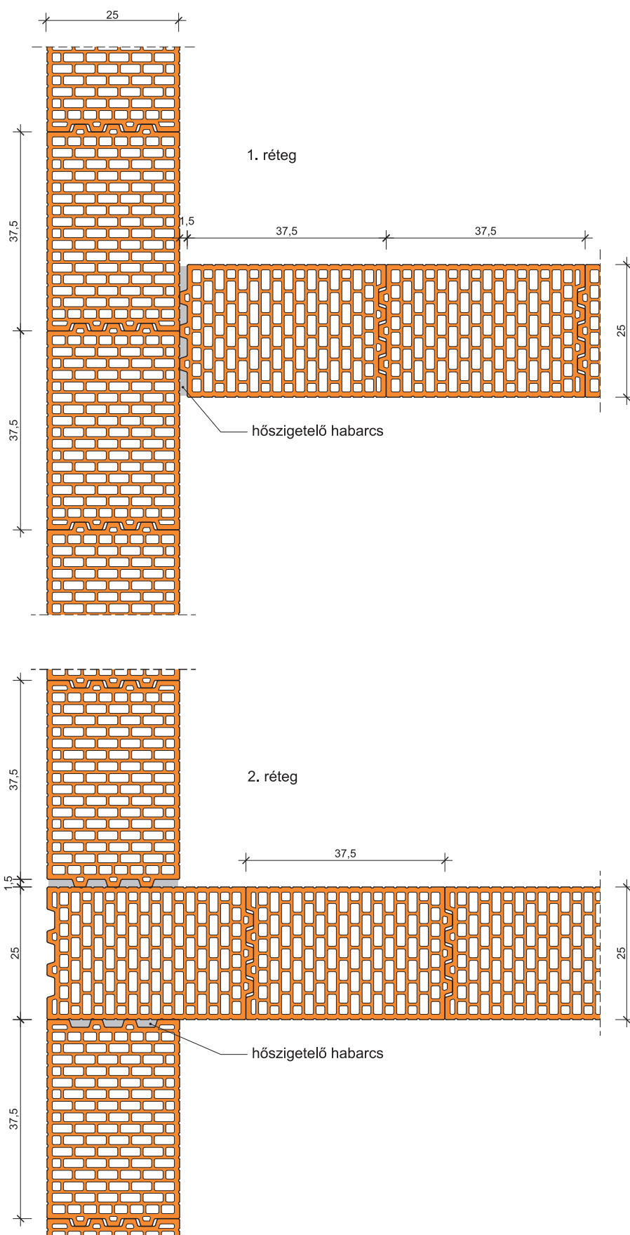
68. Falcsatlakozás: LeierPLAN 25 N+F – LeierPLAN 25 N+F / Leiertherm 25 N+F – Leiertherm 25 N+F
