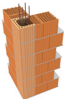
25. Leiertherm 30 U elemből készített sarokpillér
