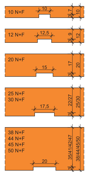
8. Függőleges falhorony legnagyobb mérete meglévő fal esetén
