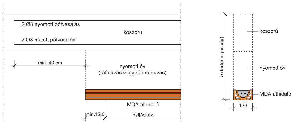
20. Tartómagasság értelmezése Leier MDA és Leier MDVA nyílásáthidalónál
