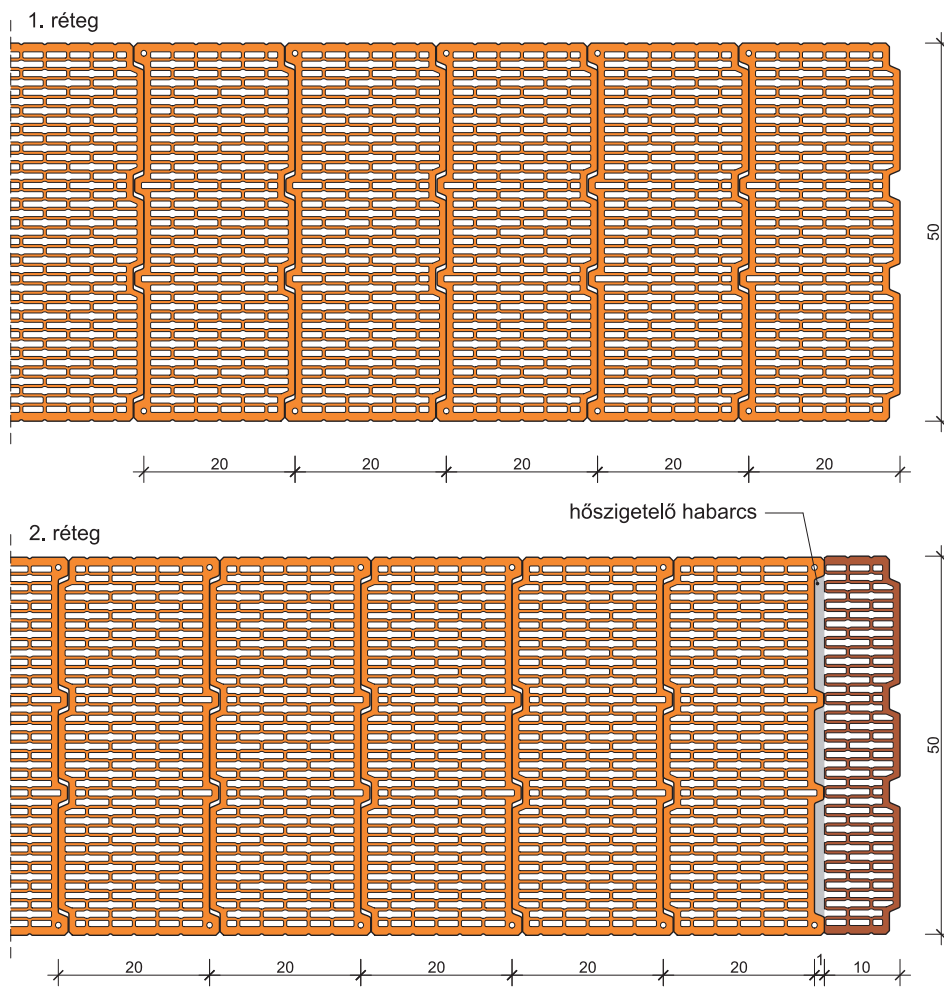
58. Falvég: LeierPLAN 50 Pro / Leiertherm 50 Pro
