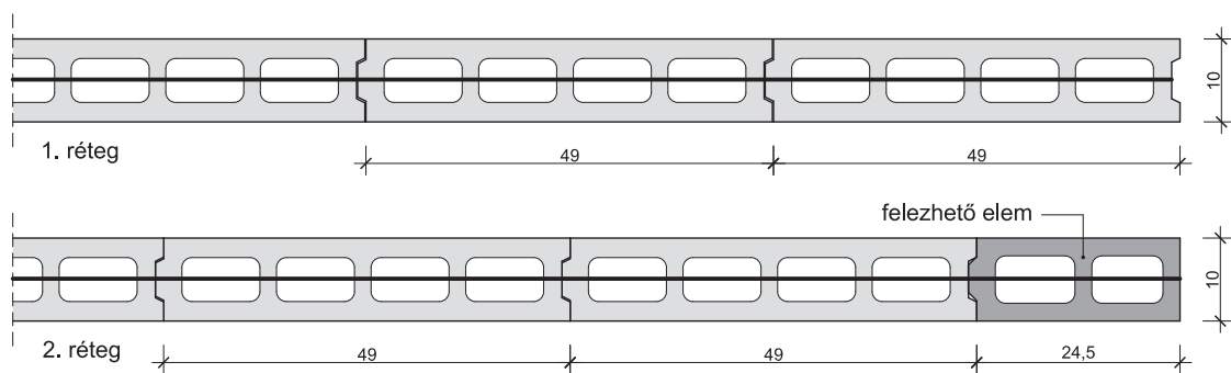
18. Falvég: Leier beton válaszfalelem VF 10
