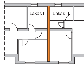
27. Lakásválasztó fal
