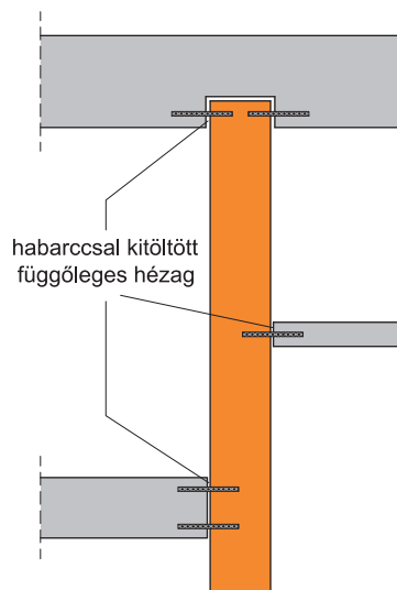
31. Bekötőszalag alkalmazása
