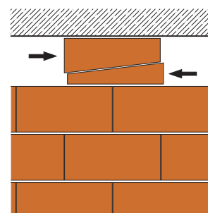
5. Válaszfal kiékelése
