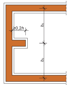
4. Pincefal geometriai méretei
