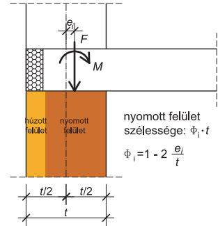
5. Külpontosság értelmezése
