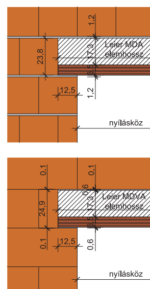
45. Méretek – Leier MDA és Leier MDVA nyílásáthidaló
