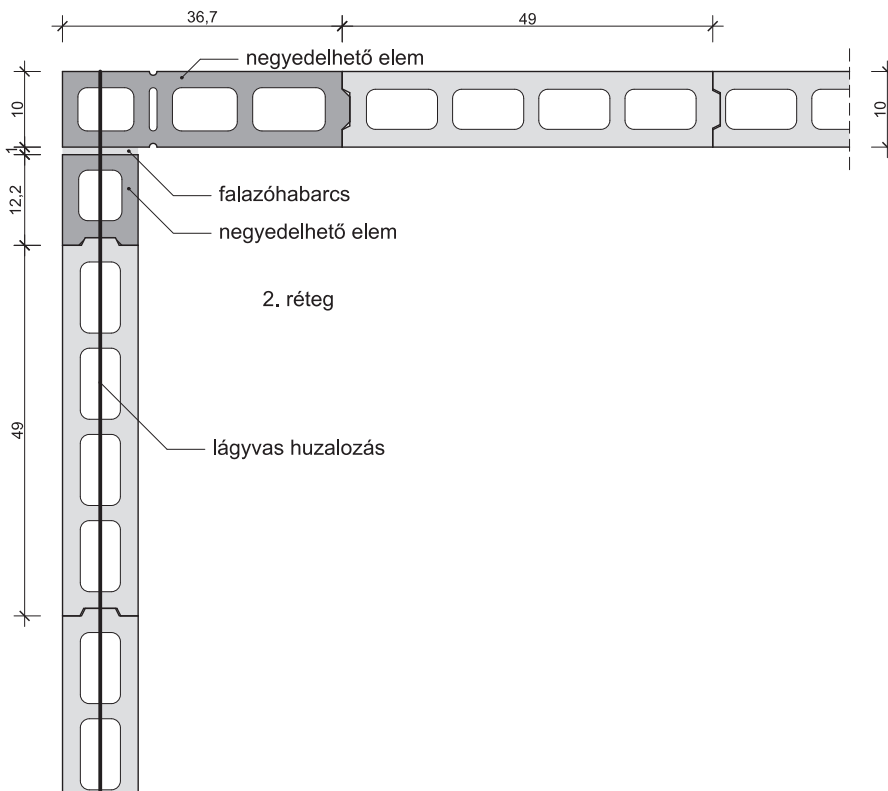
17. Falsarok: Leier beton válaszfalelem VF 10
