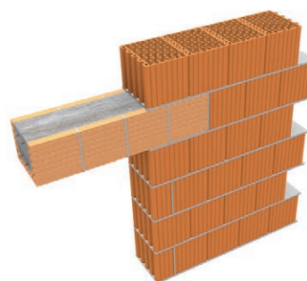
26. Leiertherm 30 U elemből készített áthidalás
