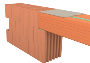
9. Leier MDE nyílásáthidaló beépítése
