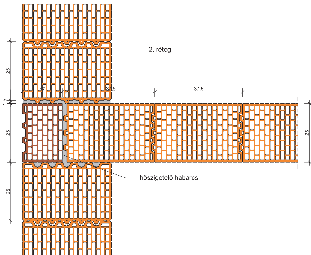
73. FalcSATlakozás: LeierPLAN 38 Pro – LeierPLAN 25 N+F / LeierPLAN 38 N+F – LeierPLAN 25 N+F Leiertherm 38 Pro – Leiertherm 25 N+F / Leiertherm 38 N+F – Leiertherm 25 N+F
