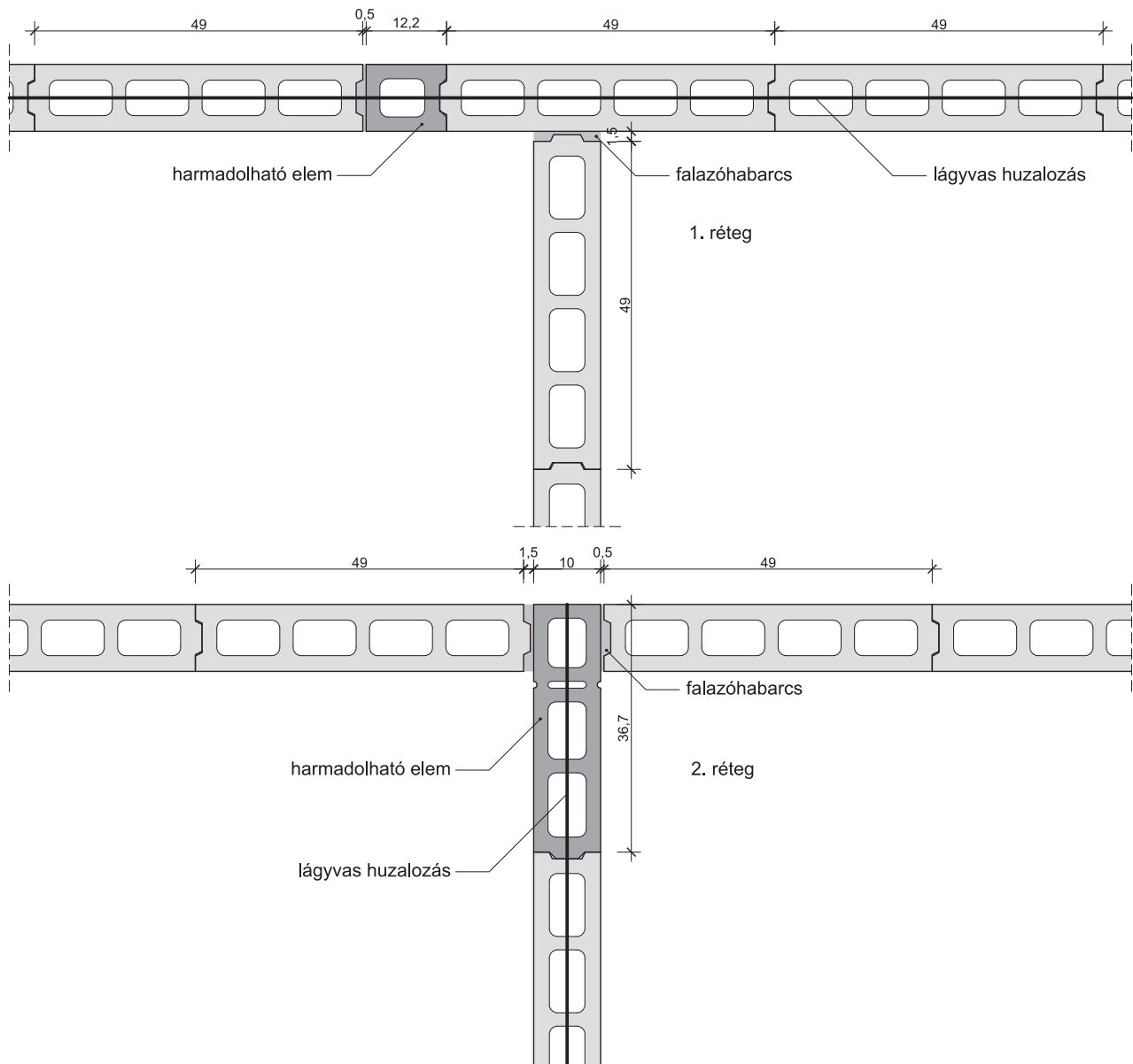
19. Falsarok: Leier beton válaszfalelem VF 10
