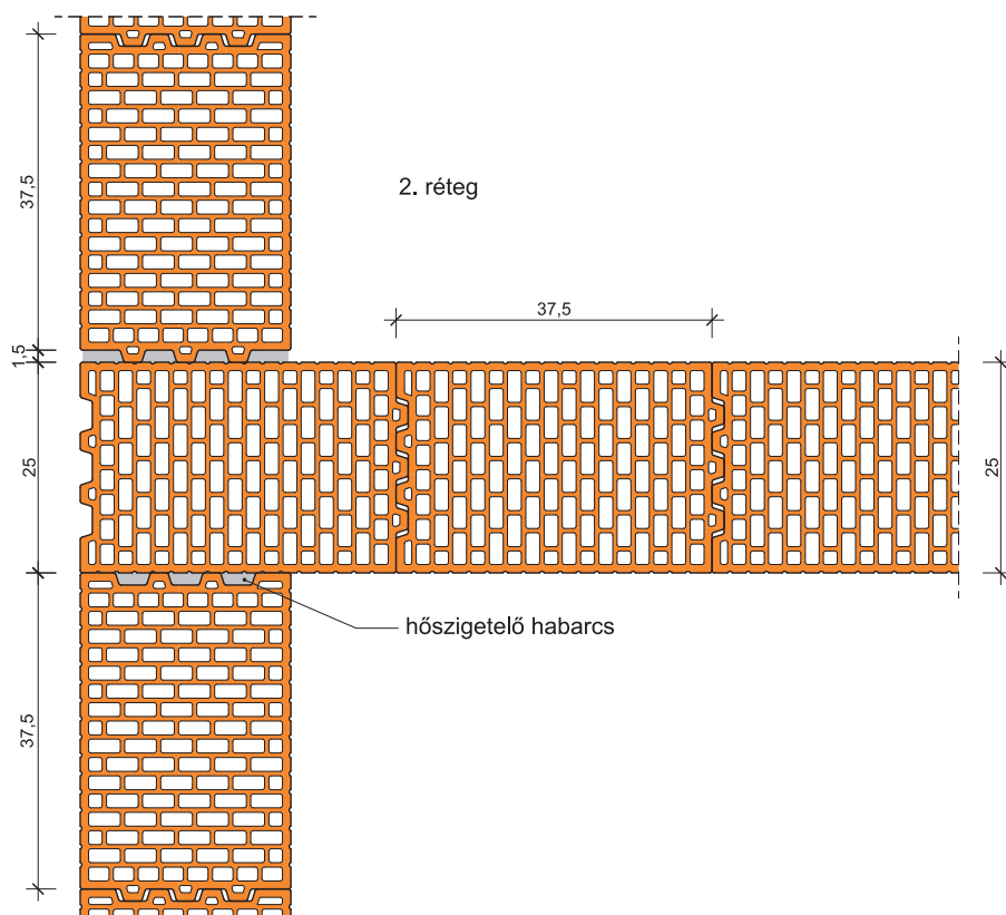
68. Falcsatlakozás: LeierPLAN 25 N+F – LeierPLAN 25 N+F / Leiertherm 25 N+F – Leiertherm 25 N+F
