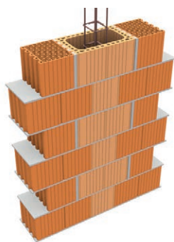
23. Leiertherm 30 U elemből készített falközi pillér - téglakötésben rakva
