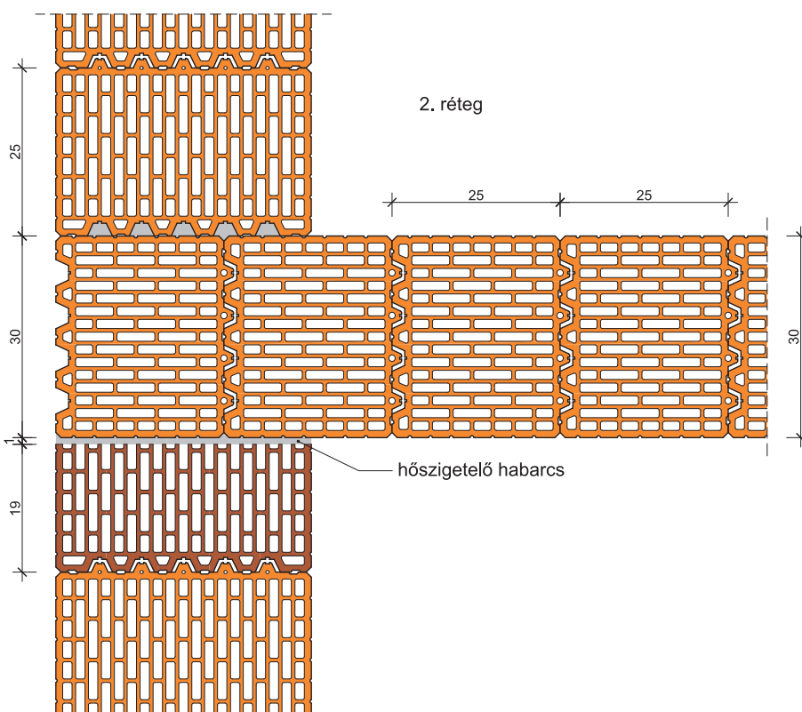
74. Falcsatlakozás: LeierPLAN 38 Pro – LeierPLAN 30 Pro / LeierPLAN 38 N+F – LeierPLAN 30 N+F Leiertherm 38 Pro – Leiertherm 30 Pro / Leiertherm 38 N+F – Leiertherm 30 N+F
