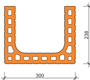
22. Leiertherm 30 U koszorúelem metszete
